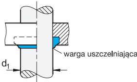
Przykład montażu
